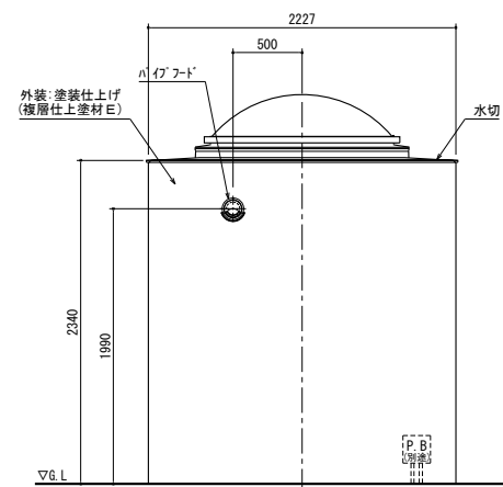
背面図
