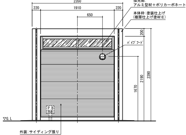
背面図
