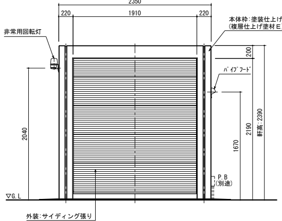
側面図
