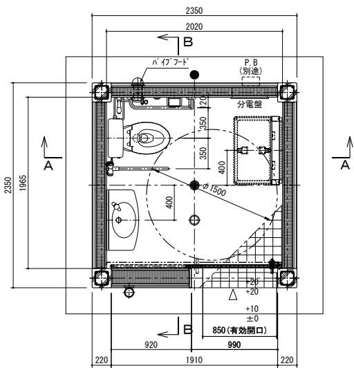
配置図 ●印: 壁上部 F I X 窓(横タイプ) 取付
