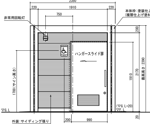
正面図
