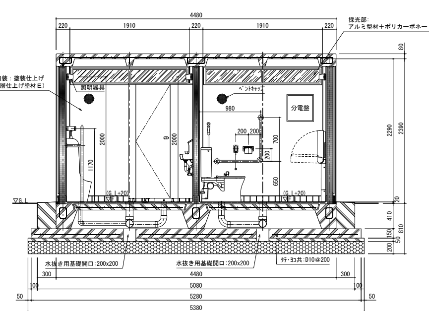
A-A 断面図
