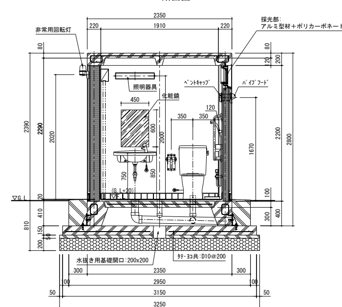
B-B 断面図
