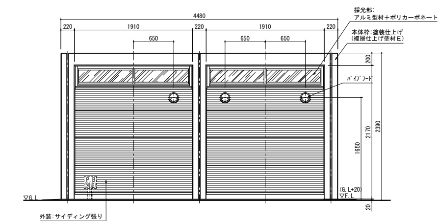
背面図
