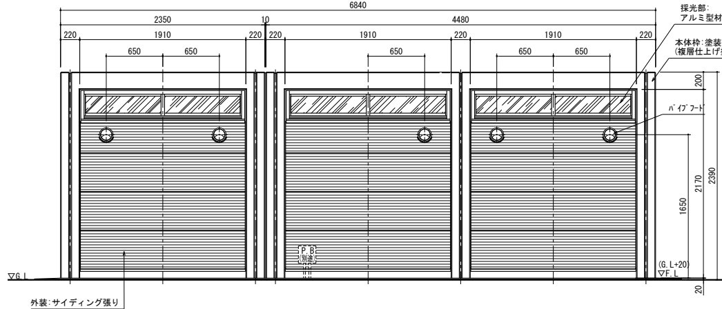
背面図
