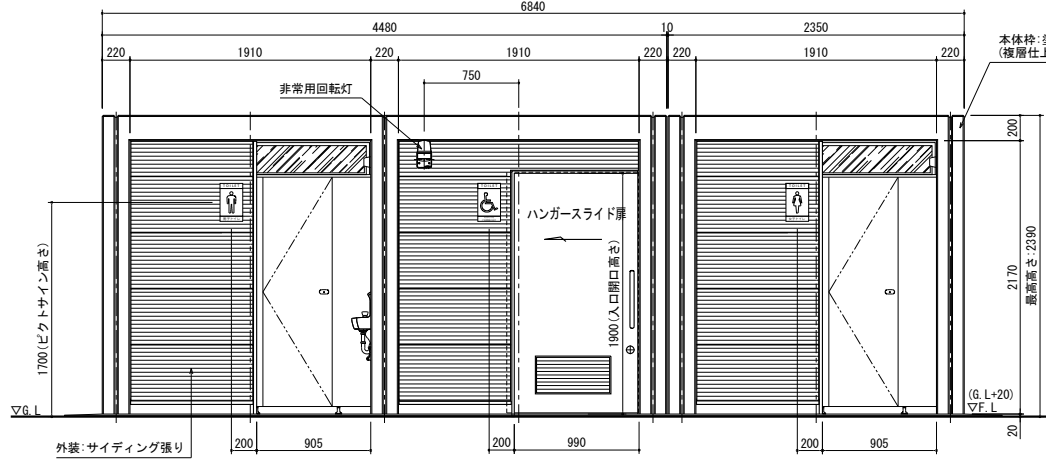
正面図
