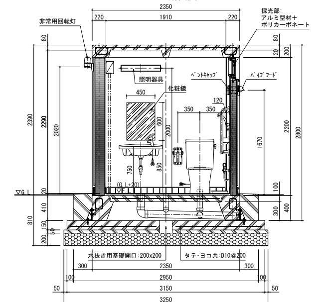
B-B 断面図
