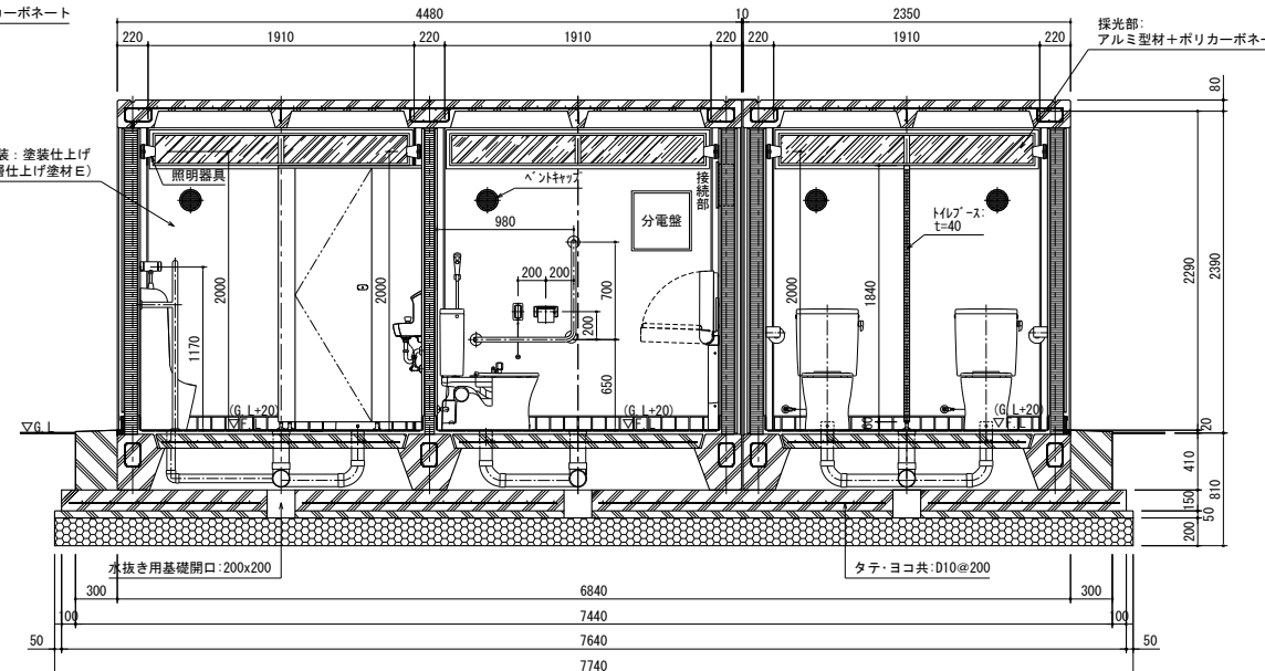
A-A 断面図
