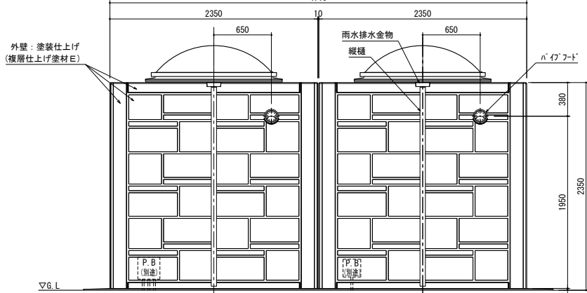
背面図
