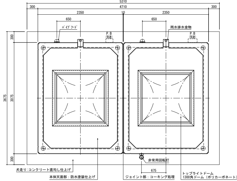
平面図
