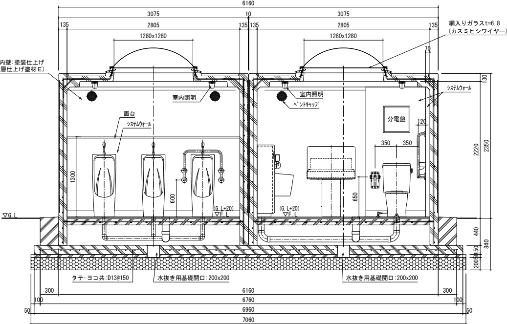
A-A 断面図
