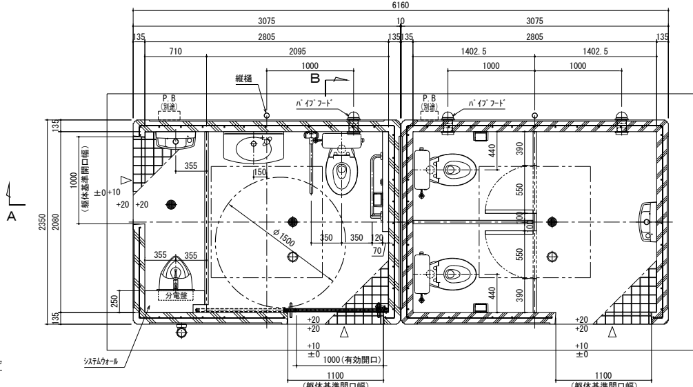
配置図
