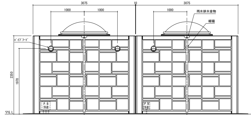
背面図
