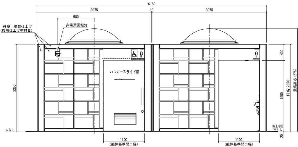
正面図
