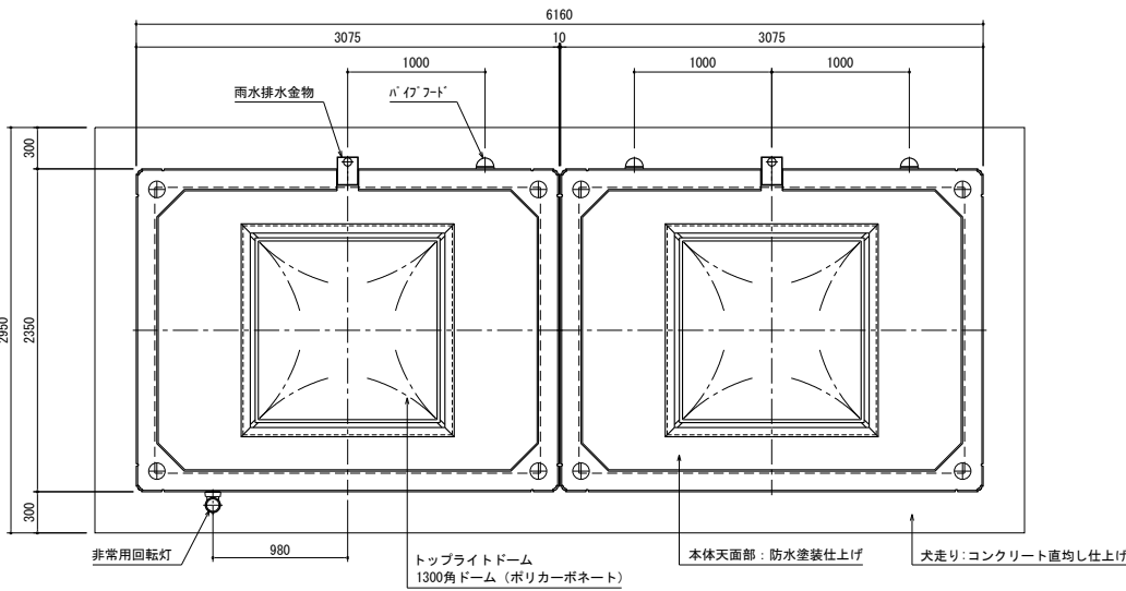
平面図
