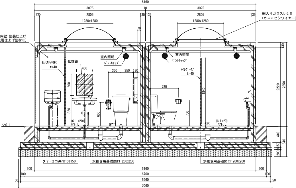
A-A 断面図
