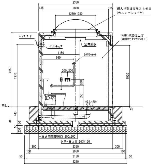
B-B 断面図
