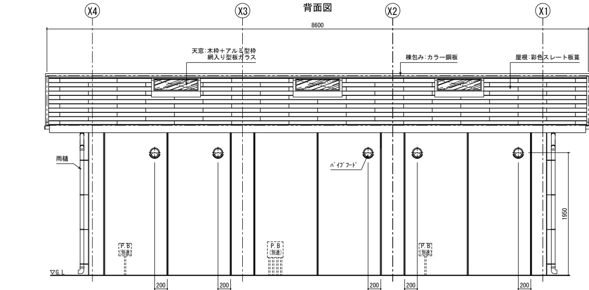
背面図
