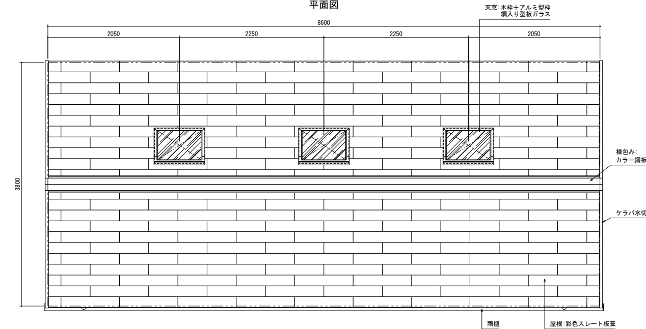
平面図
