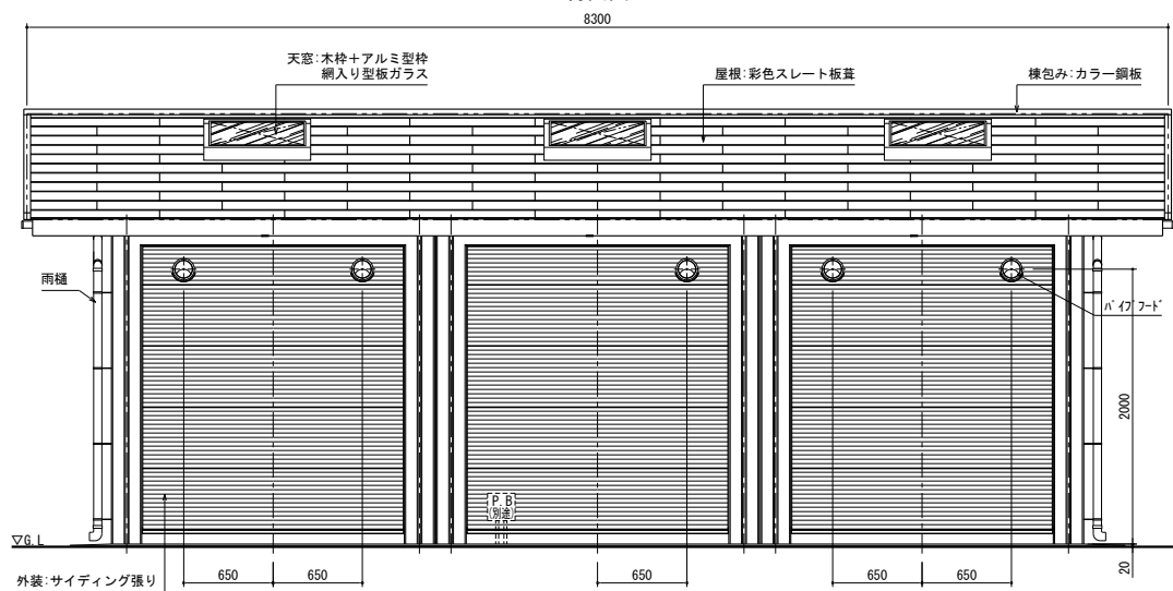
背面図
