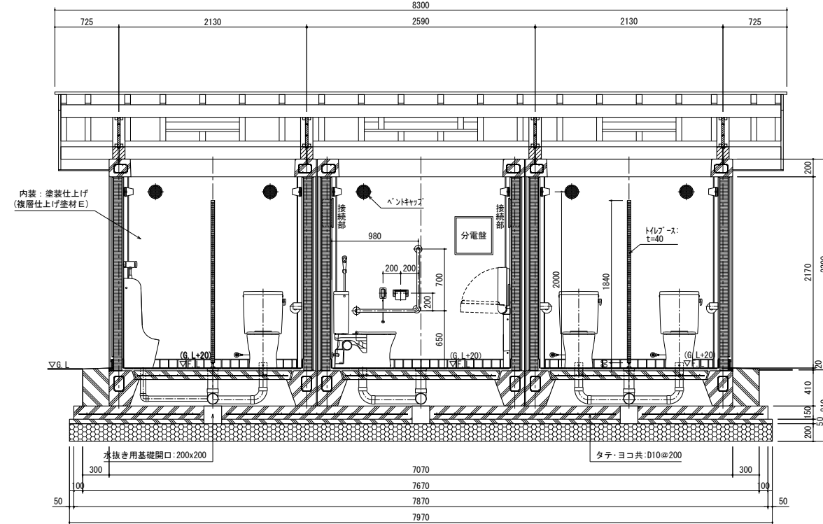
A-A 断面図
