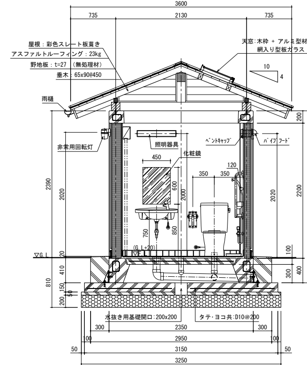
B-B 断面図
