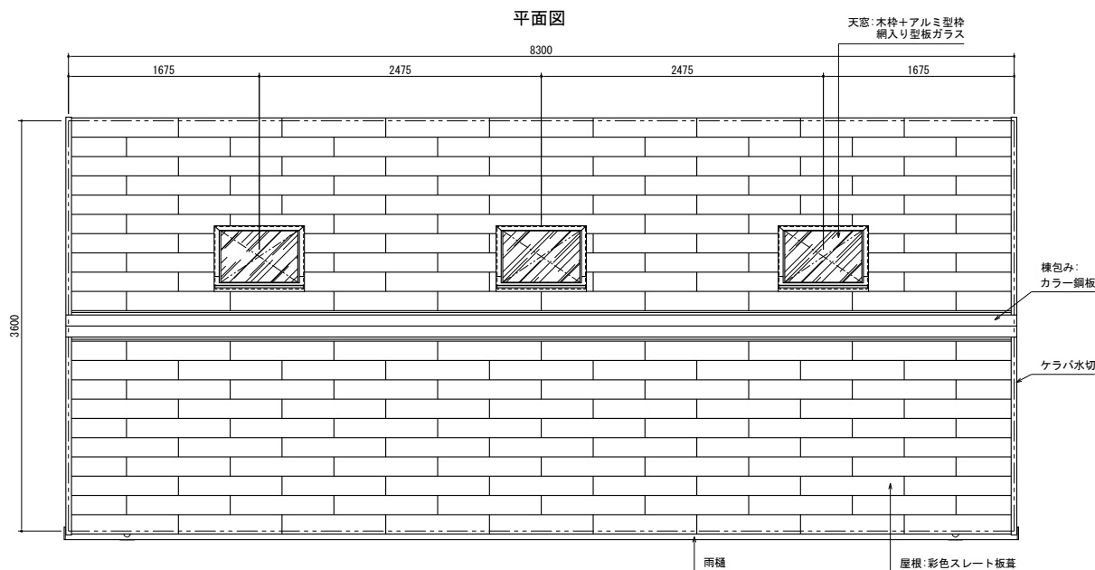
平面図
