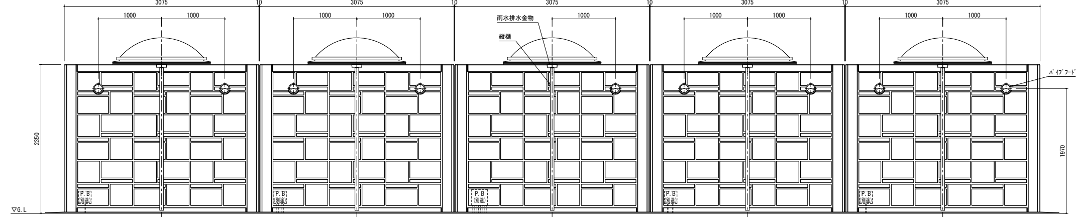
背面図
