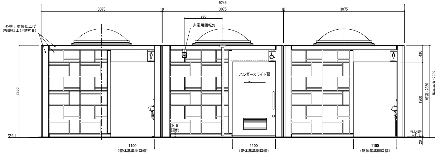
正面図
