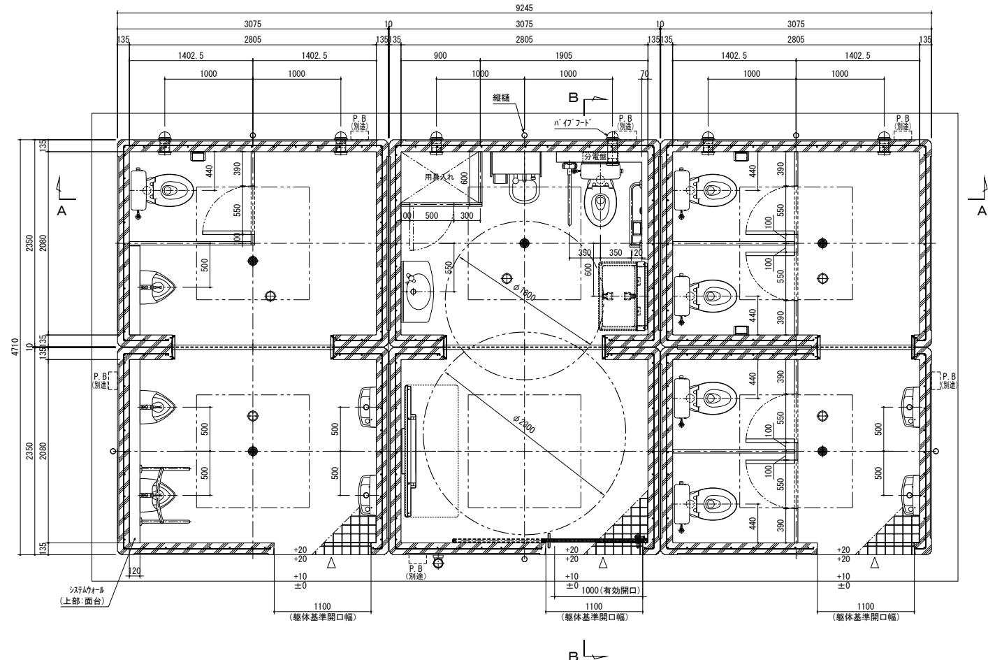
配置図
