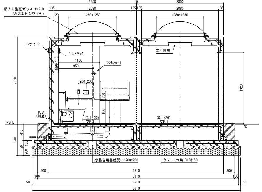
B-B 断面図
