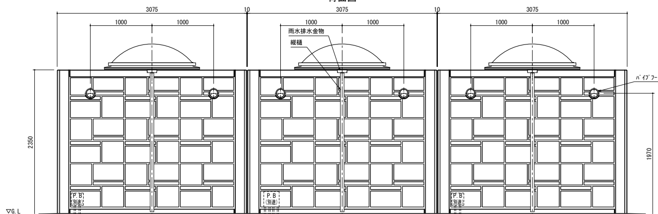
背面図
