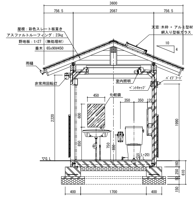
B-B 断面図
