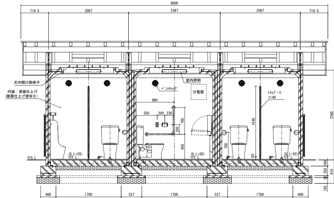
A-A 断面図
