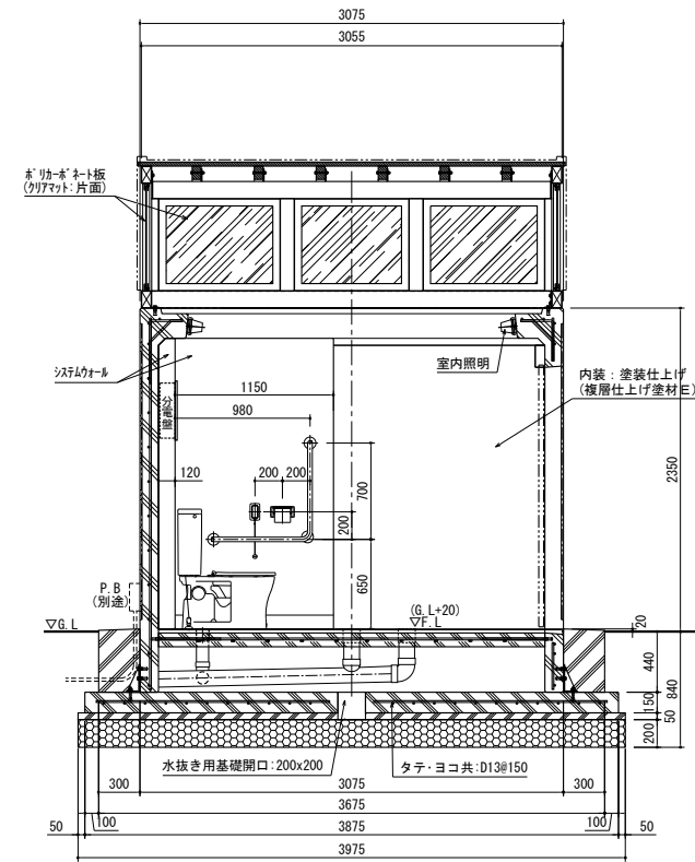
B-B 断面図
