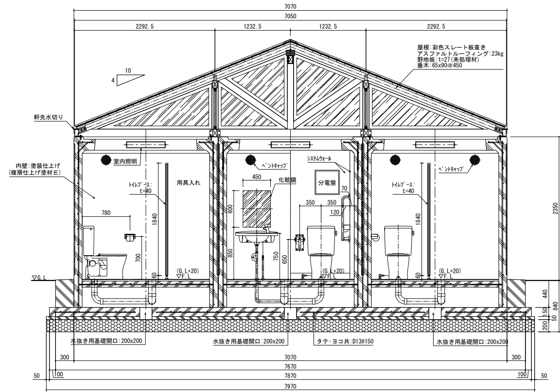
A-A 断面図
